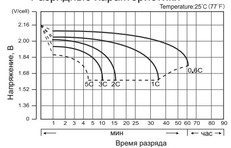
Разрядные характеристики
