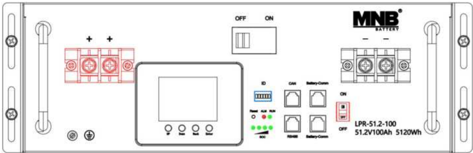
Рисунок 7-4. Схема панели
