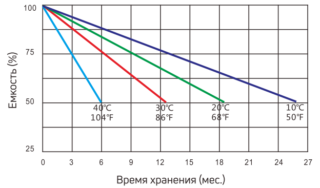
Показатели саморазряда
