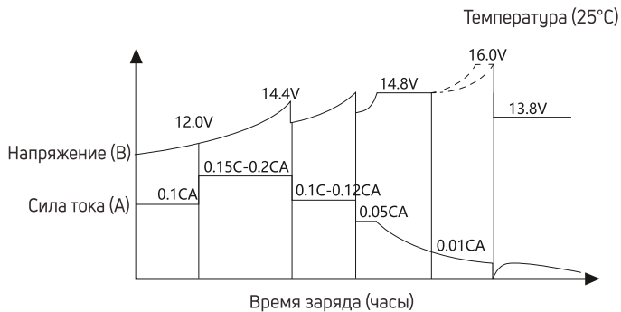
Характеристики заряда
